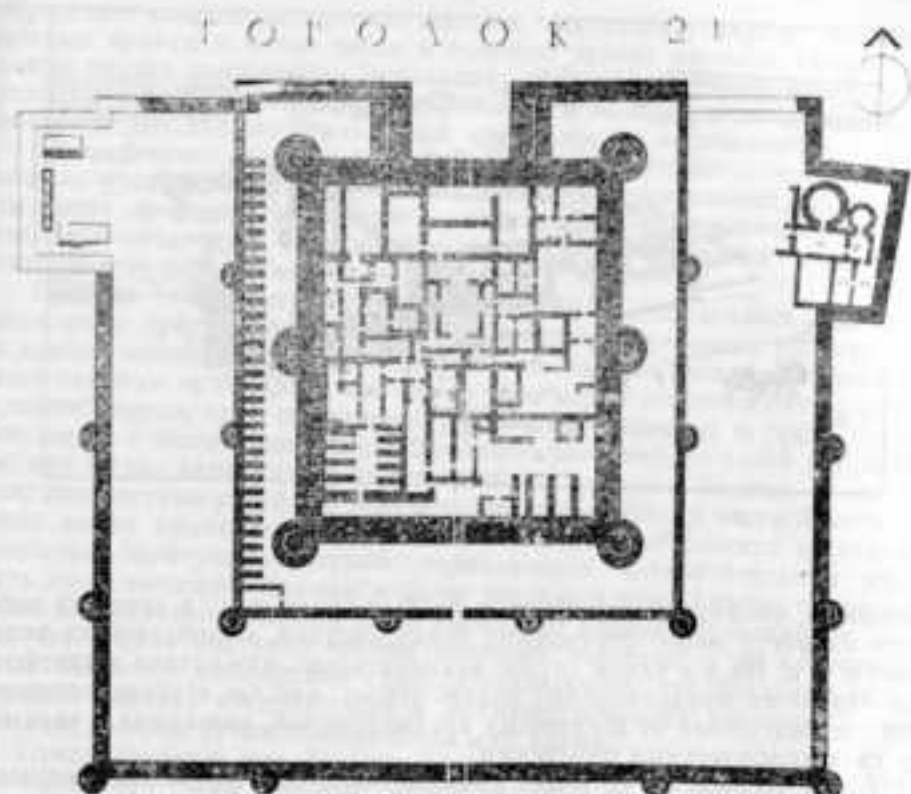
Рис. 35. Тоголок 21. План первого, основного периода храма.
