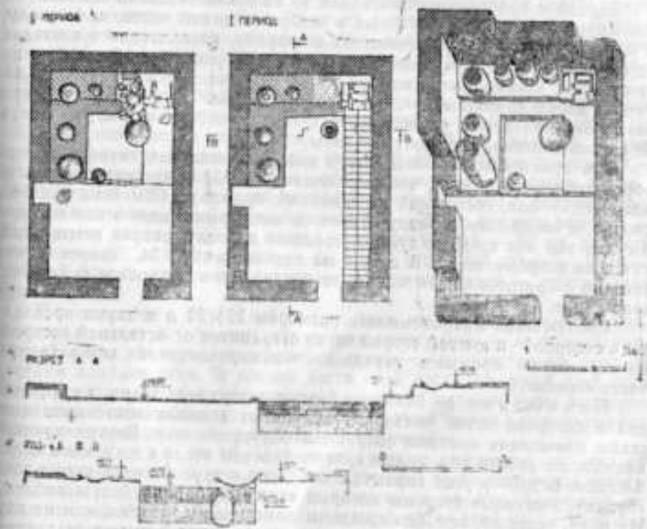
Рис. 20. Табл. 21. Помещение № 34. План и реконструкция.
