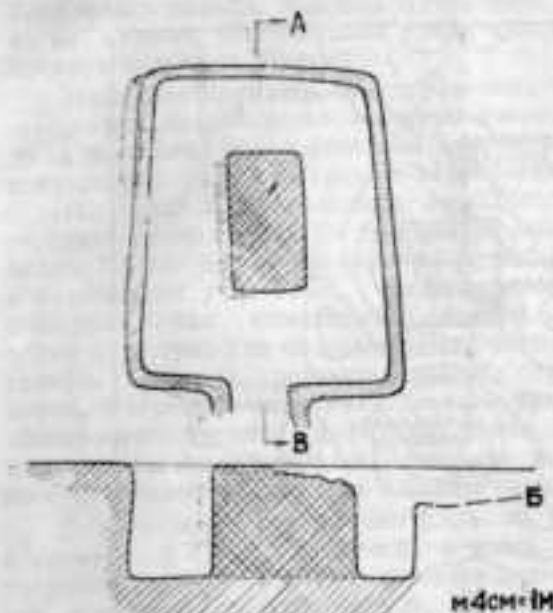
Рис. 5. Гонур 1. Гончарная печь.
